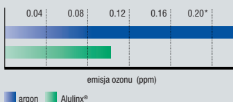
Średnia emisja ozonu przy ręcznym spawaniu metodą MIG blach ze stopu AlMg5 (przenoszenie natryskowe)
