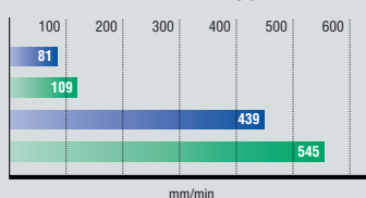
Średnia prędkość spawania ręcznego metodą MIG oraz TIG blachy 10mm ze stopu aluminium
